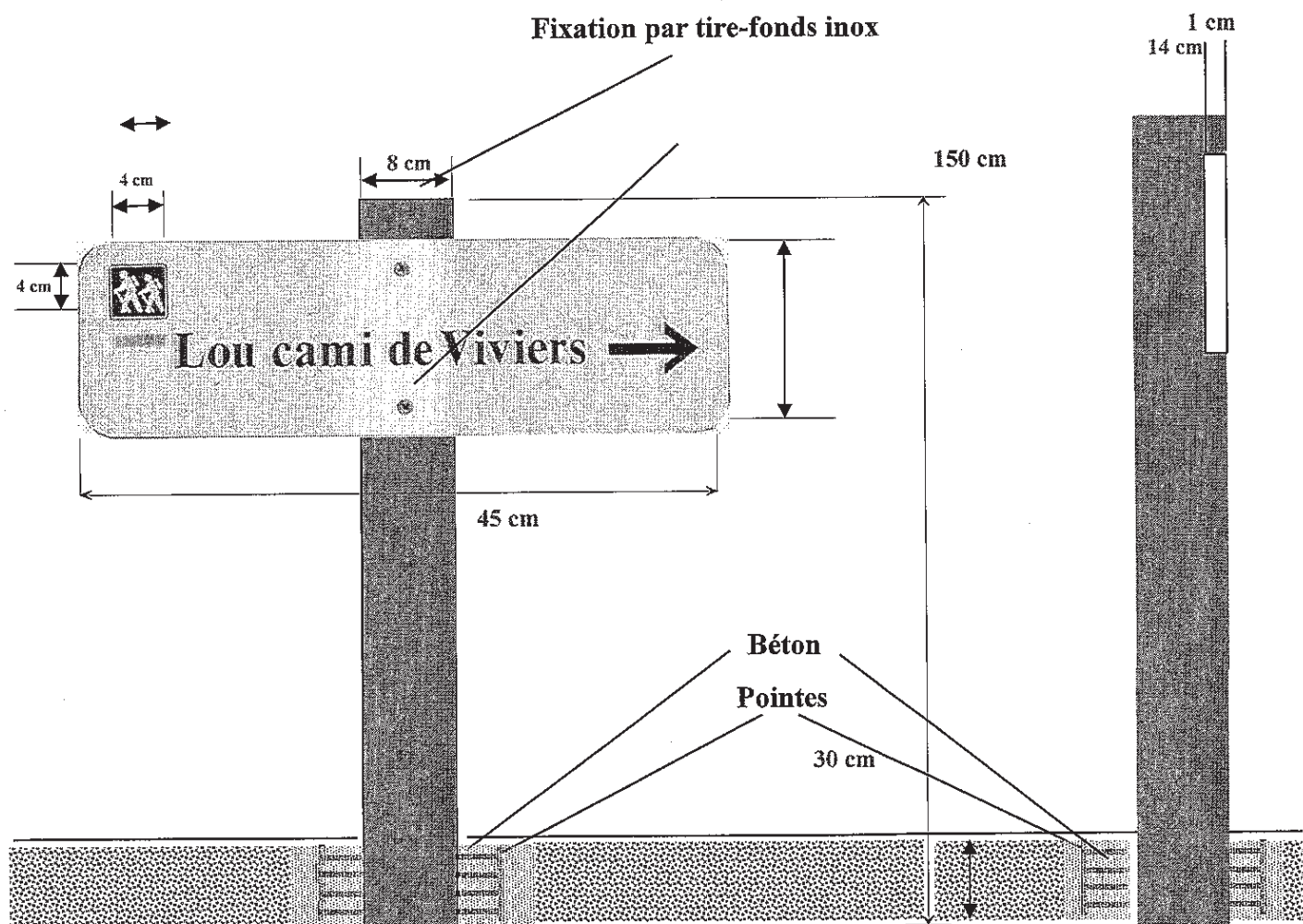
Vue de profil avec encastrement du panneau directionne
